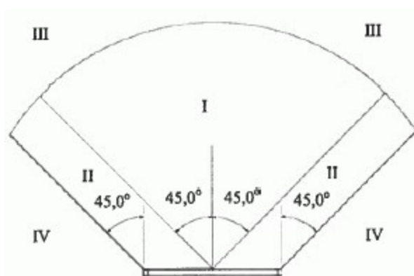
Рис. 1. Зонирование учебных помещений по комфорту зрительного восприятия от ЭСО коллективного использования.
