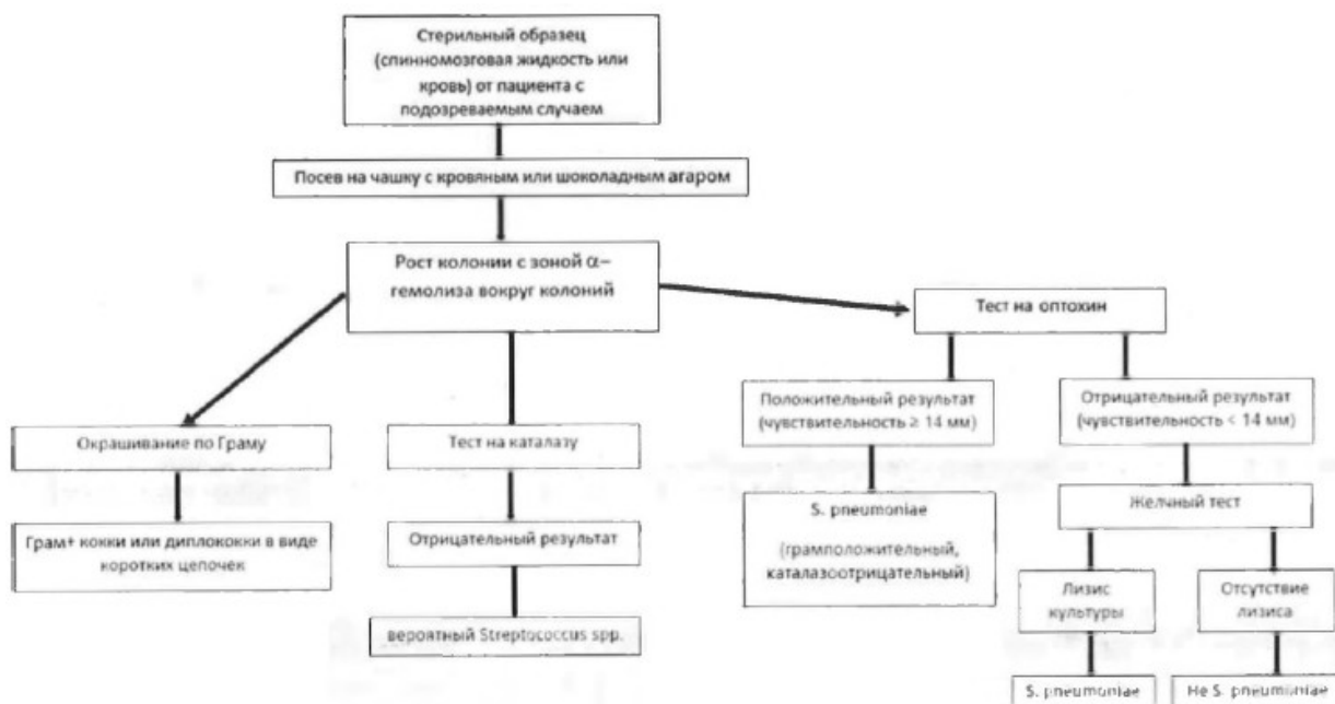
Схема обнаружения H. influenzae в клиническом материале
