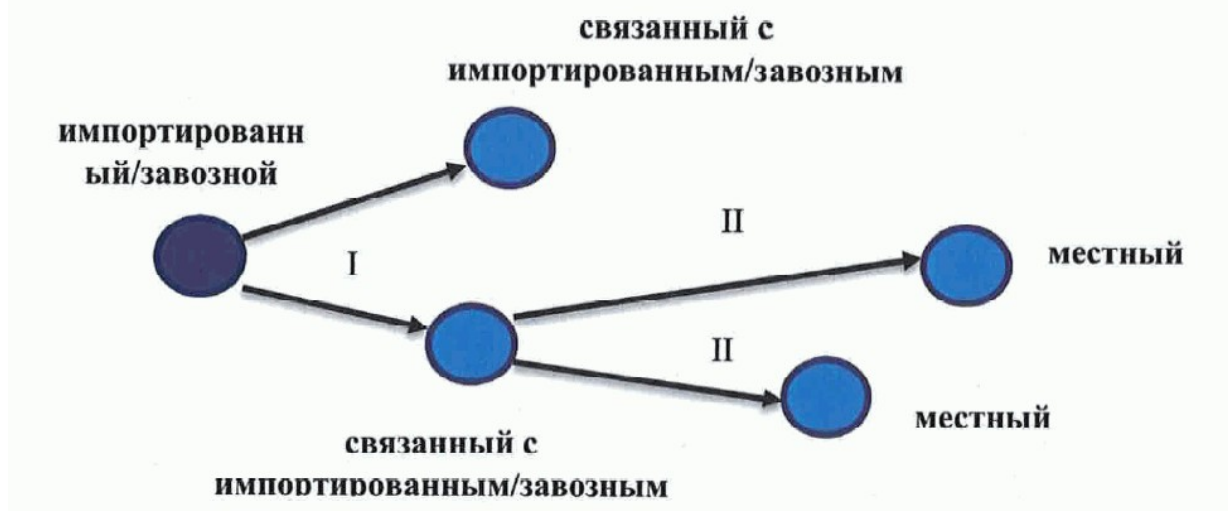
Рисунок 2. Схема вторичного распространения кори на уровне второго поколения воспроизводства инфекции
