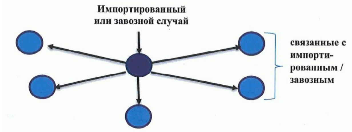
Рисунок 1. Схема вторичного распространения кори на уровне первого поколения воспроизводства инфекции
