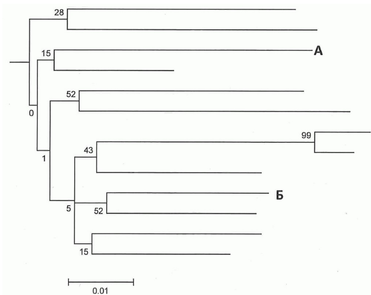
Рис. 2. Филогенетическое дерево 2
