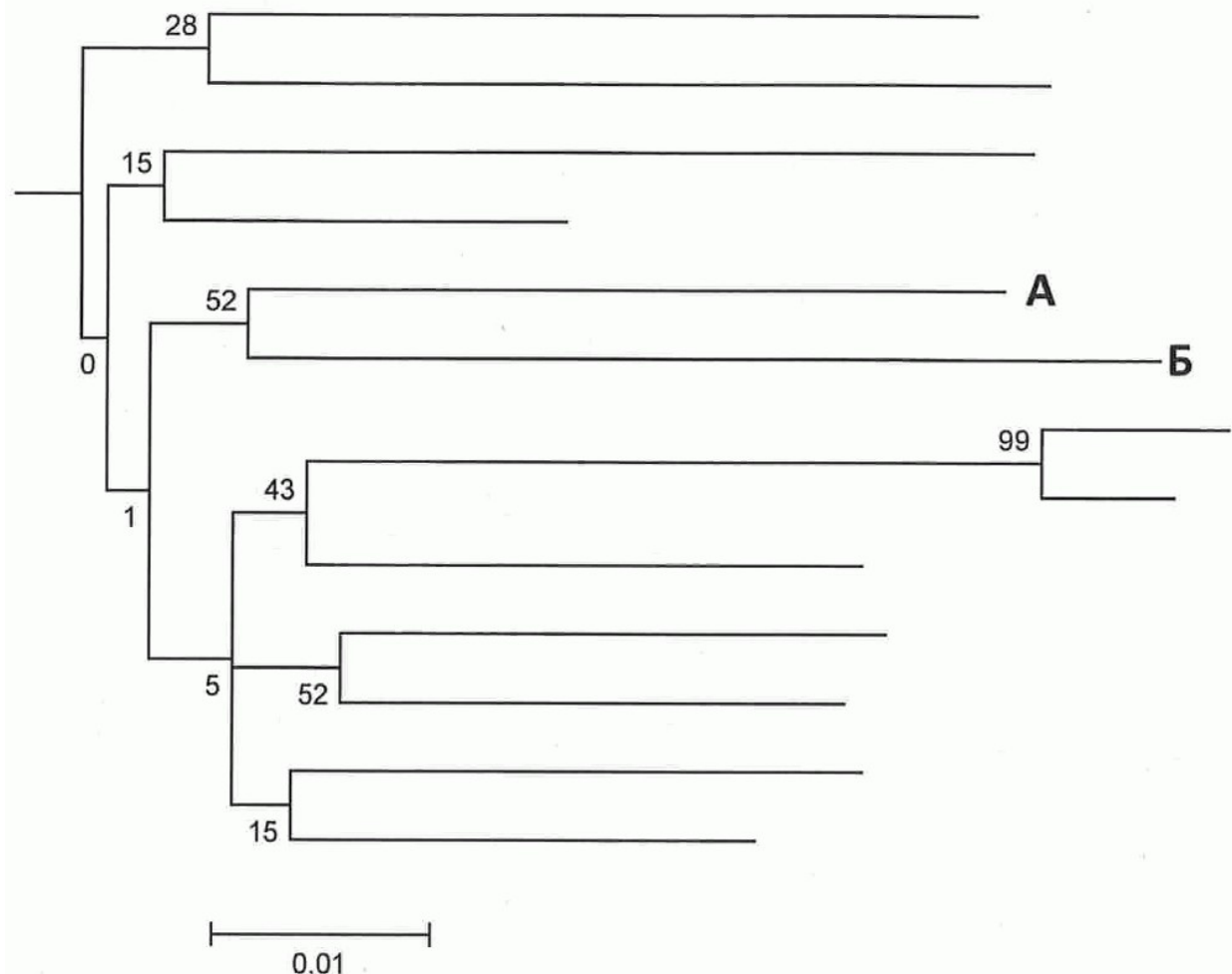
Рис. 5. Филогенетическое дерево 5
