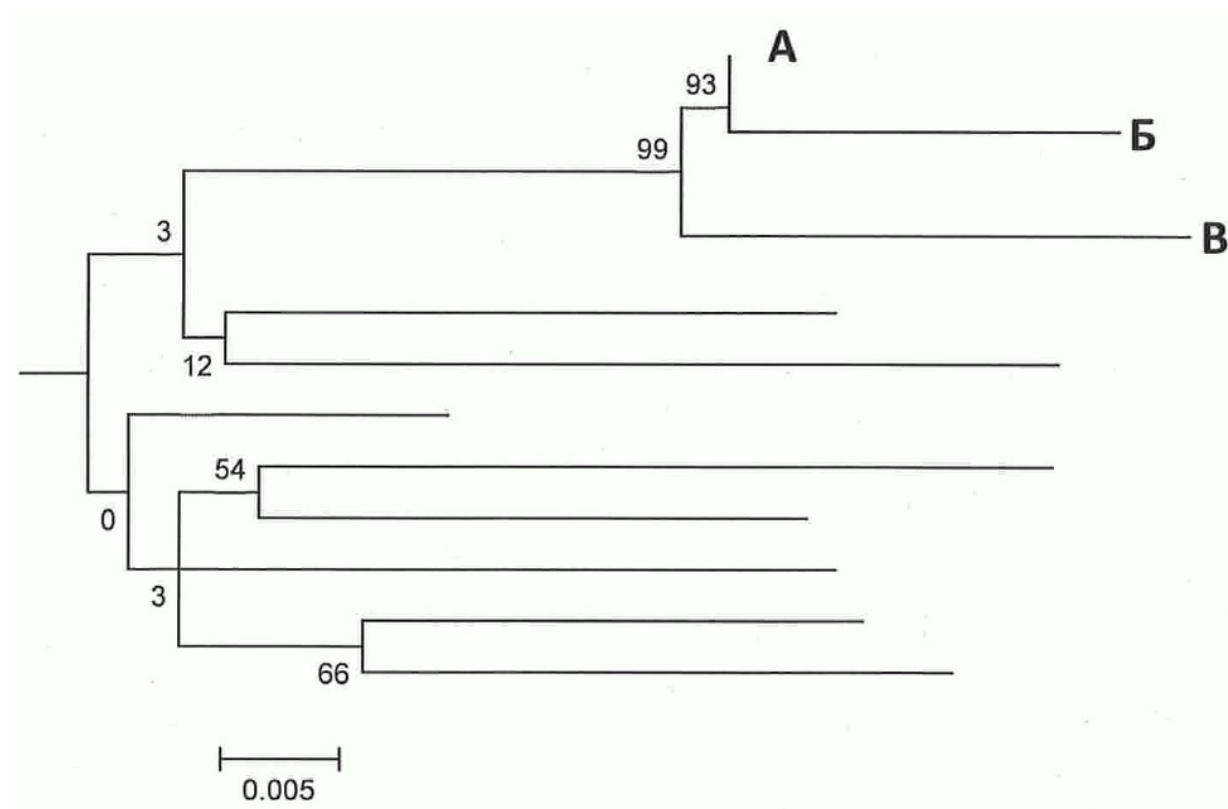
Рис. 4. Филогенетическое дерево 4
