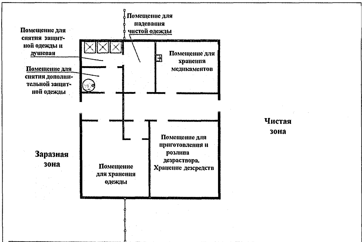
Блок санитарного пропуска медперсонала
