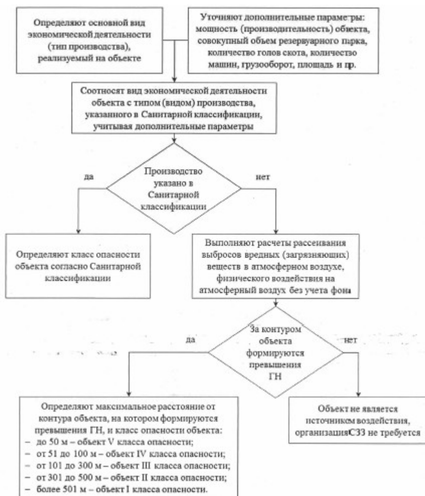
Рис. 1. Алгоритм определения класса опасности объекта
